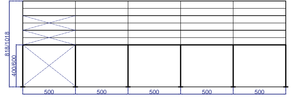
YAN GÖRÜNÜŞ
