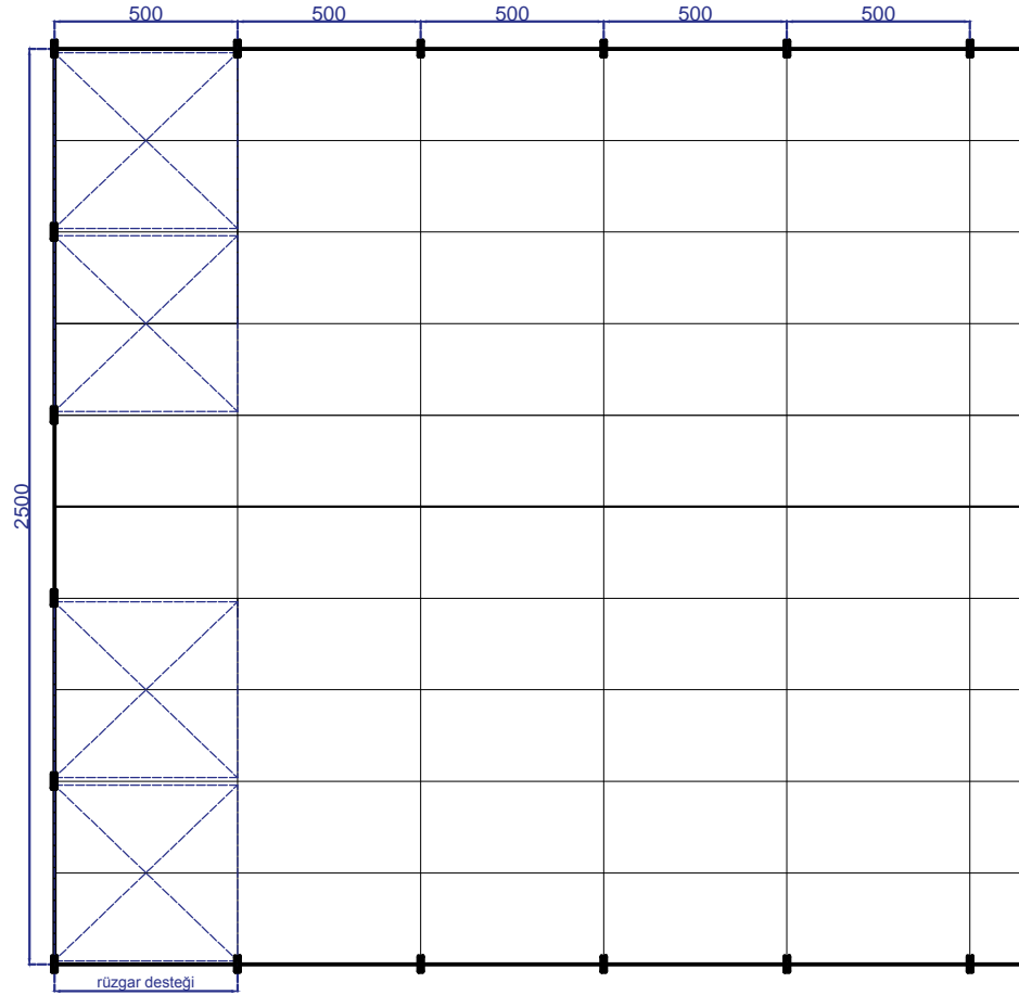
TEPE GÖRÜNÜŞÜ
