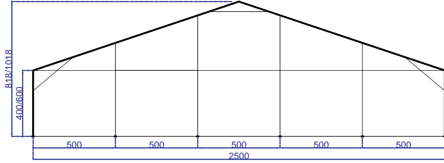
ÖN GÖRÜNÜŞ
