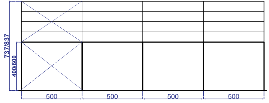
YAN GÖRÜNÜŞ
