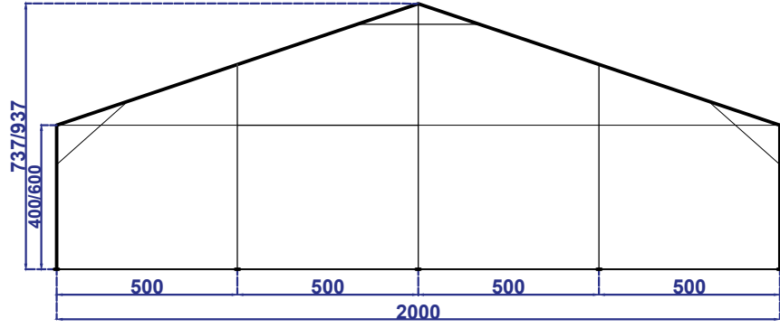
ÖN GÖRÜNÜŞ
