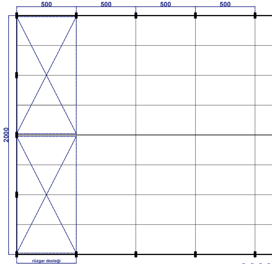
TEPE GÖRÜNÜŞÜ
